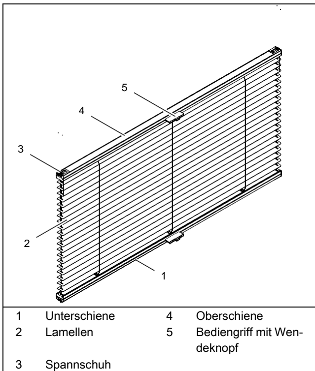
Abb. 1: Teileübersicht Jalousie Luna
