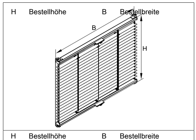
Abb. 3: Maßskizze Jalousie Luna (geklebte Ausführung)
