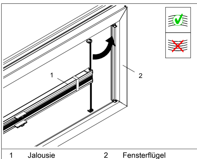
Abb. 6: Jalousie in Fensterflügel einsetzen
